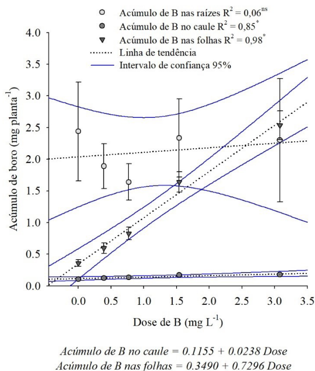
Figura 4. Acúmulo de B nas folhas, caules e raízes em função das doses de B.
