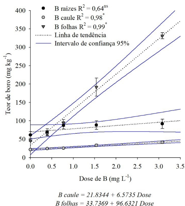
Figura 1. Teor de B nas folhas, caule e raízes em função das doses de B.
