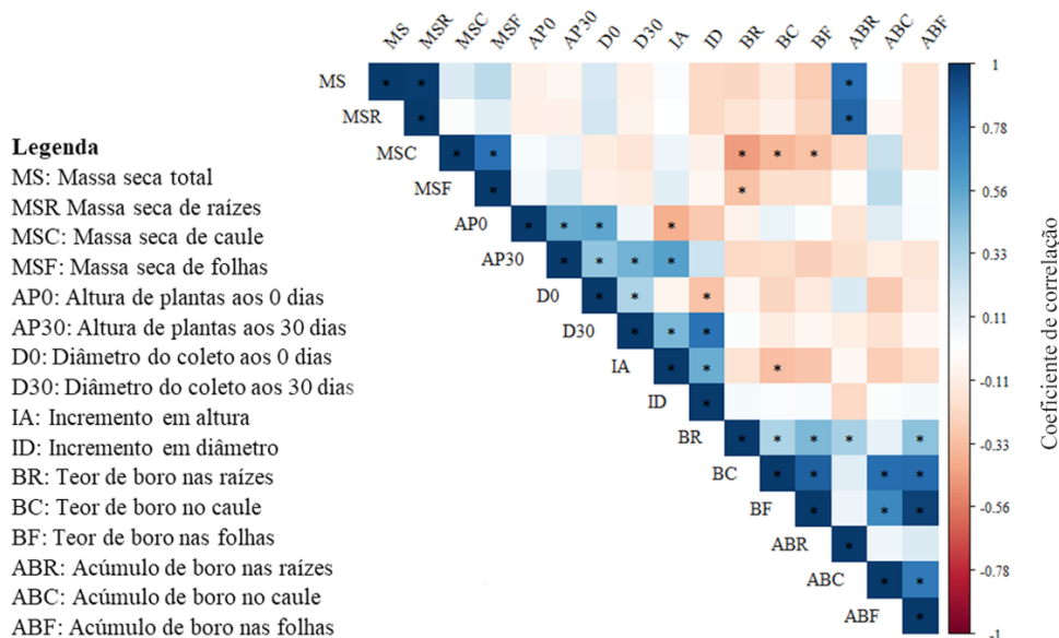
Figura 6. Análise de correlação de Pearson entre as variáveis analisadas para o eucalypto submetido a doses e formas de aplicação de B; * significativo a 0,05 de probabilidade.
